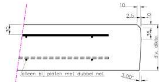
Doorsnede A
