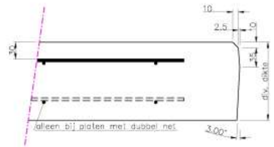
Doorsnede A
