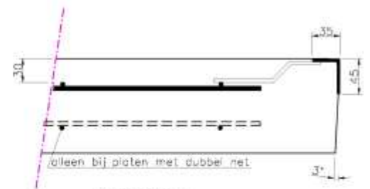
Doorsnede A
